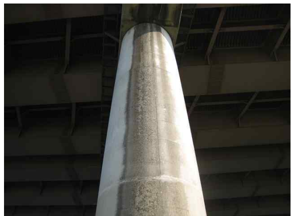
P5 배수관 위치불량-교각 누수오염의 원인(범물방향)
